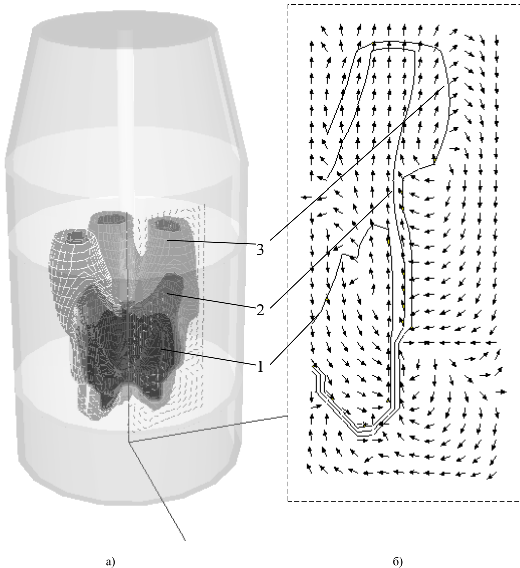
Рис. 1. Динаміка продування конвертерної вани із використанням 5-соплової фурми на початку запалювання: а) поверхні рівної об'ємної концентрації газової фази (1 - 0,75; 2 - 0,5; 3 - 0,25); б) поле напрямків швидкостей та ізолінії об'ємної концентрації газової фази для осьового перерізу однієї лунки;
