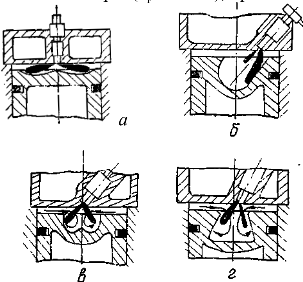
Рис. 4.12. Нерозділені камери згоряння: а—типу «Гесельман»; б—типу «Дойтц»; в—типу ЯМЗ; з—типу ЦНДДІ
