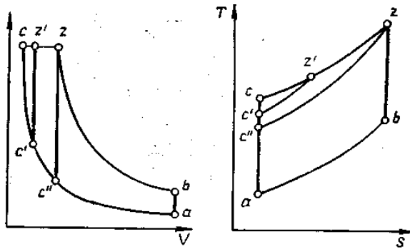
Рис. 2.4. Порівняння трьох циклів при однакових максимальних тисках і температурах у координатах p-V і T-s —const теж буде більший, а для циклу при V=\text{const} —найменший. Змішаний цикл займає проміжне місце.
