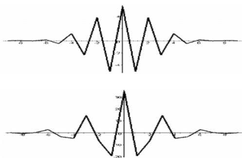
Рис. 2. Всплесковые функции биортогональной пары
