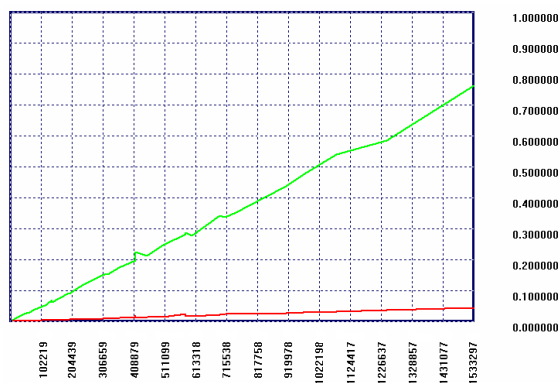
Рис. 3. Время декодирования с использованием каскадной схемы и предложенного алгоритма.
