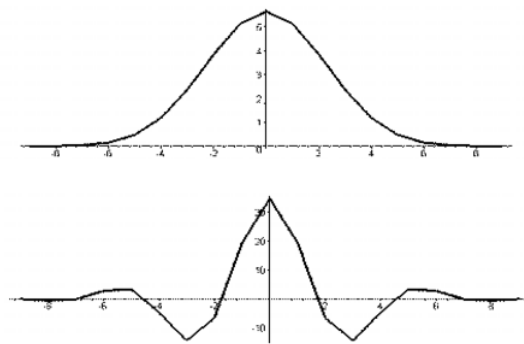
Рис. 1. Базисные функции биортогональной пары и соответствующих всплесковых функций
