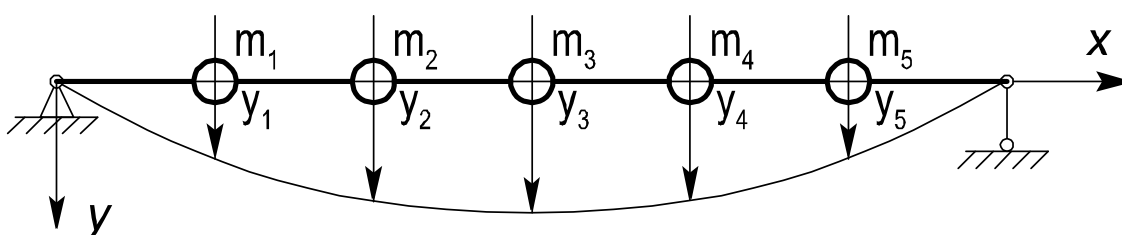
Рис. 3.1. Розрахункова схема балки з зосередженими масами
