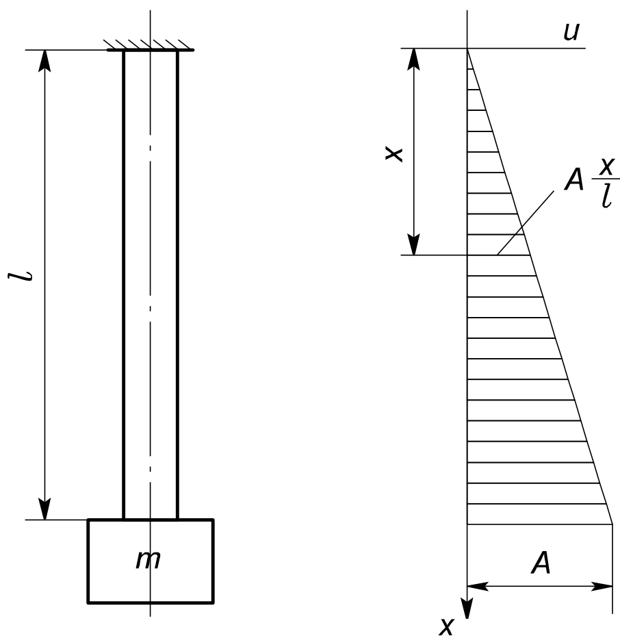
Рис. 3.3. Розрахункова схема стрижня з зосередженою масою
