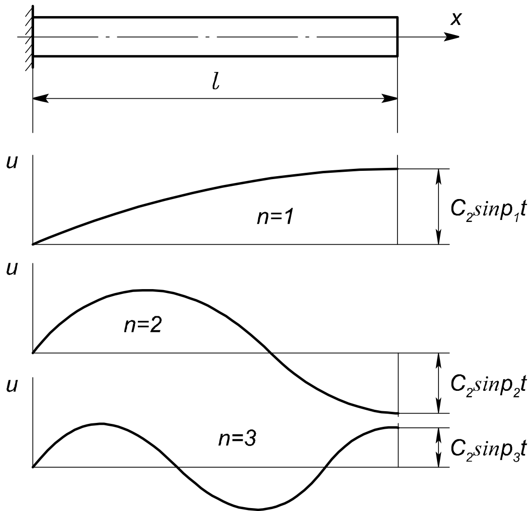
Рис. 2.4. Форми коливань стрижня
