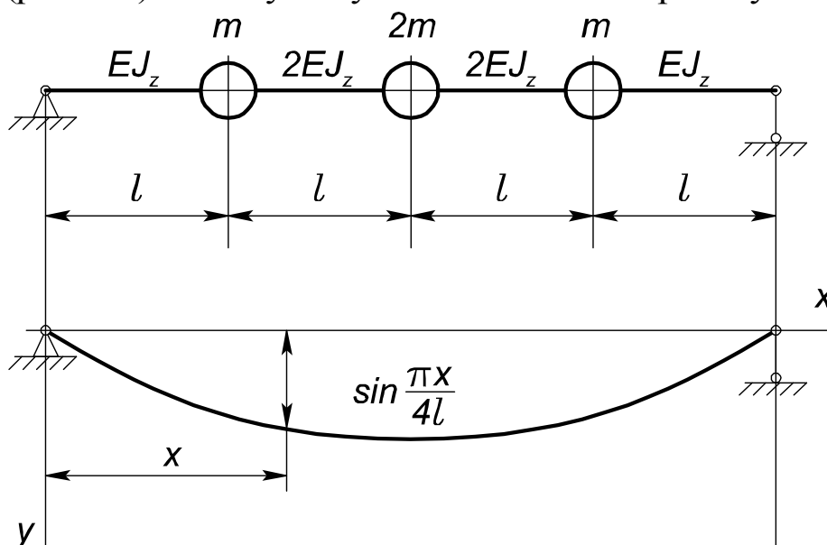
Рис. 3.2. Розрахункова схема балки з зосередженими масами
