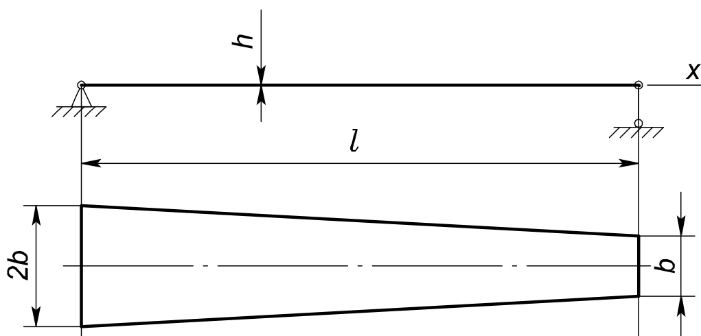
Рис. 3.4. Розрахункова схема балки з перемінними перетинами
