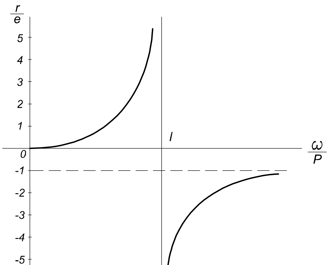
Рис. 5.3. Розташування характерних точок вала в залежності від співвідношення \omega/p .
