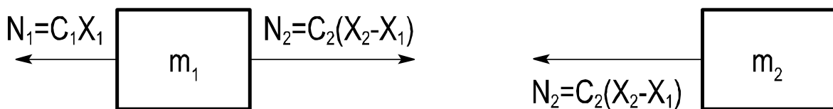
Рис. 1.2. Розрахункова схема двомасової системи до прямого способу
