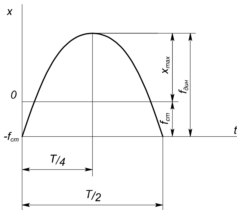
Рис. 4.4. Графік руху приєднаної маси при вертикальному поздовжньому ударі
