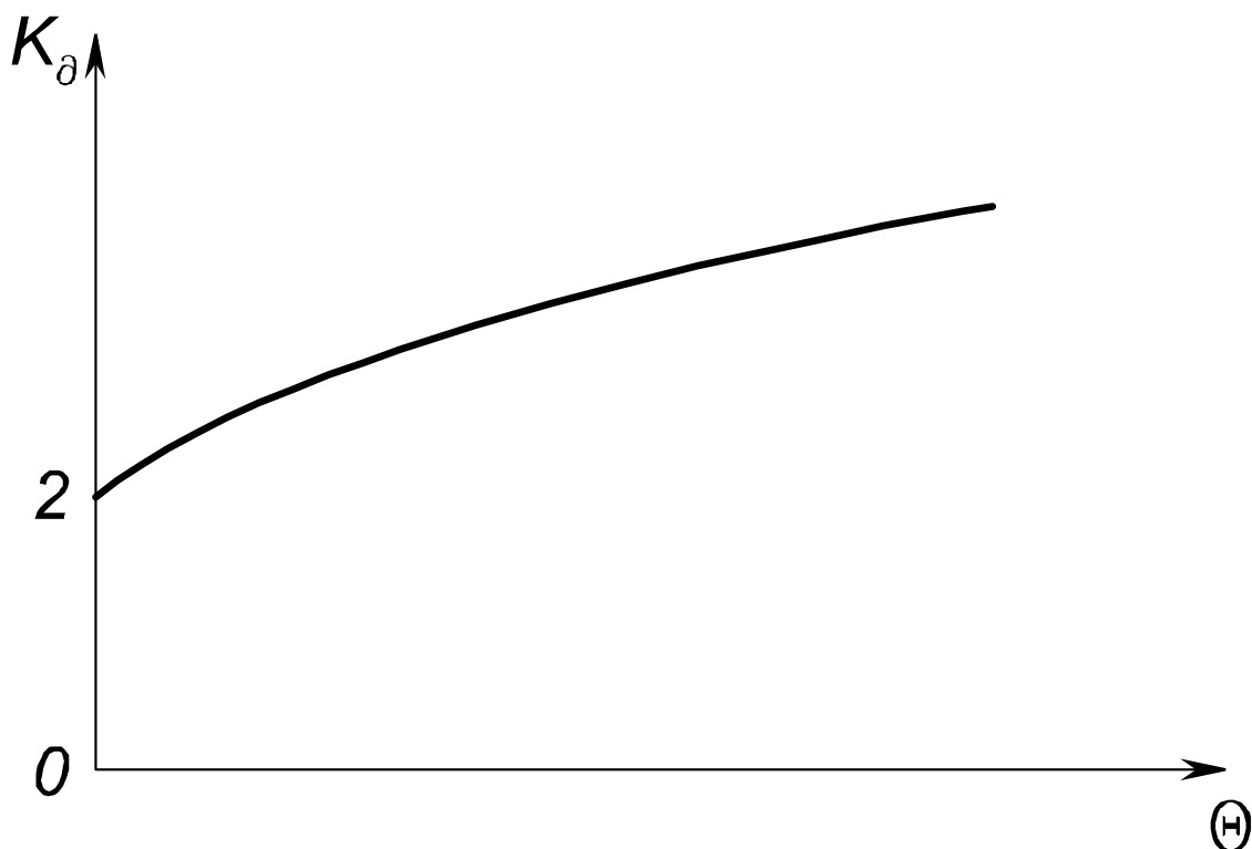
Рис. 5.11. Залежність коефіцієнтів динамічності від зазору у валопроводі
