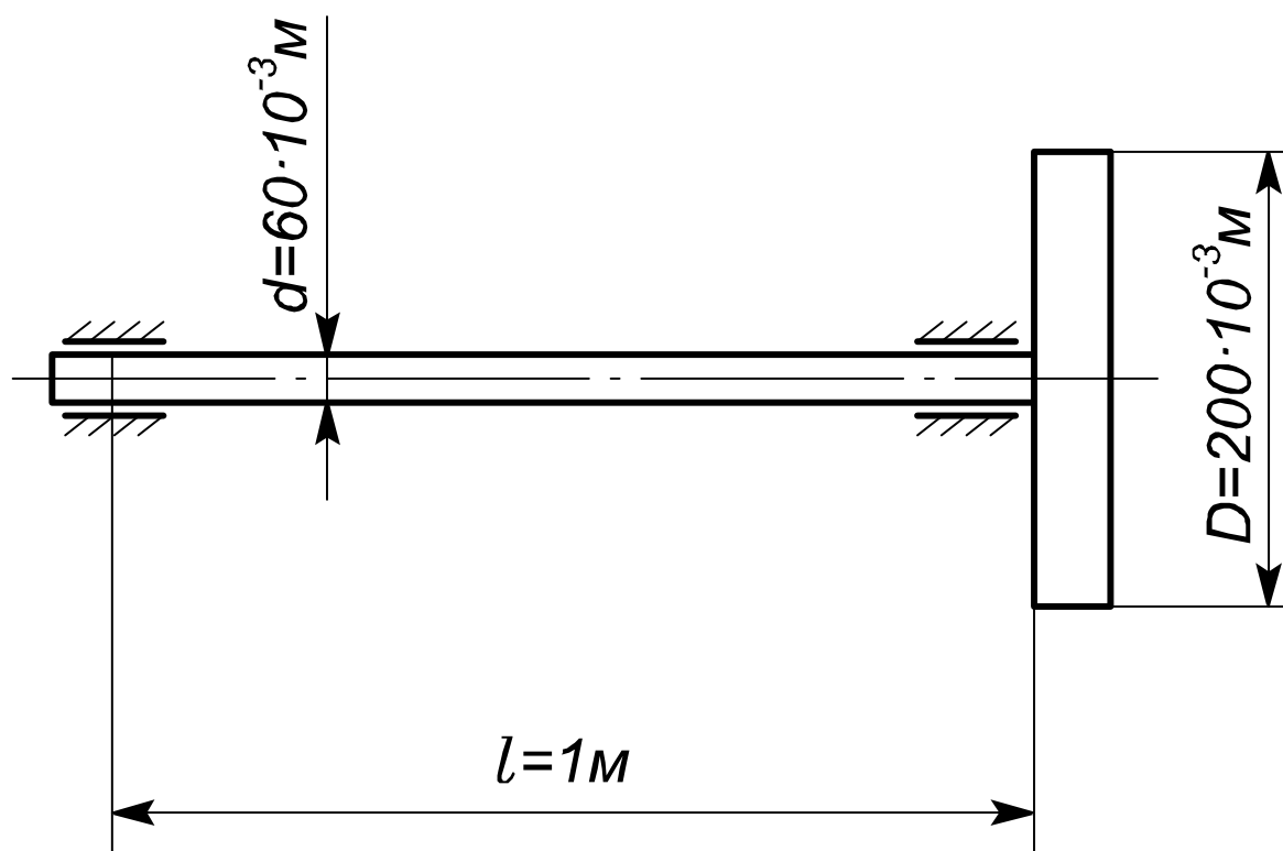
Рис. 4.6. Розрахункова схема валу з маховиком
