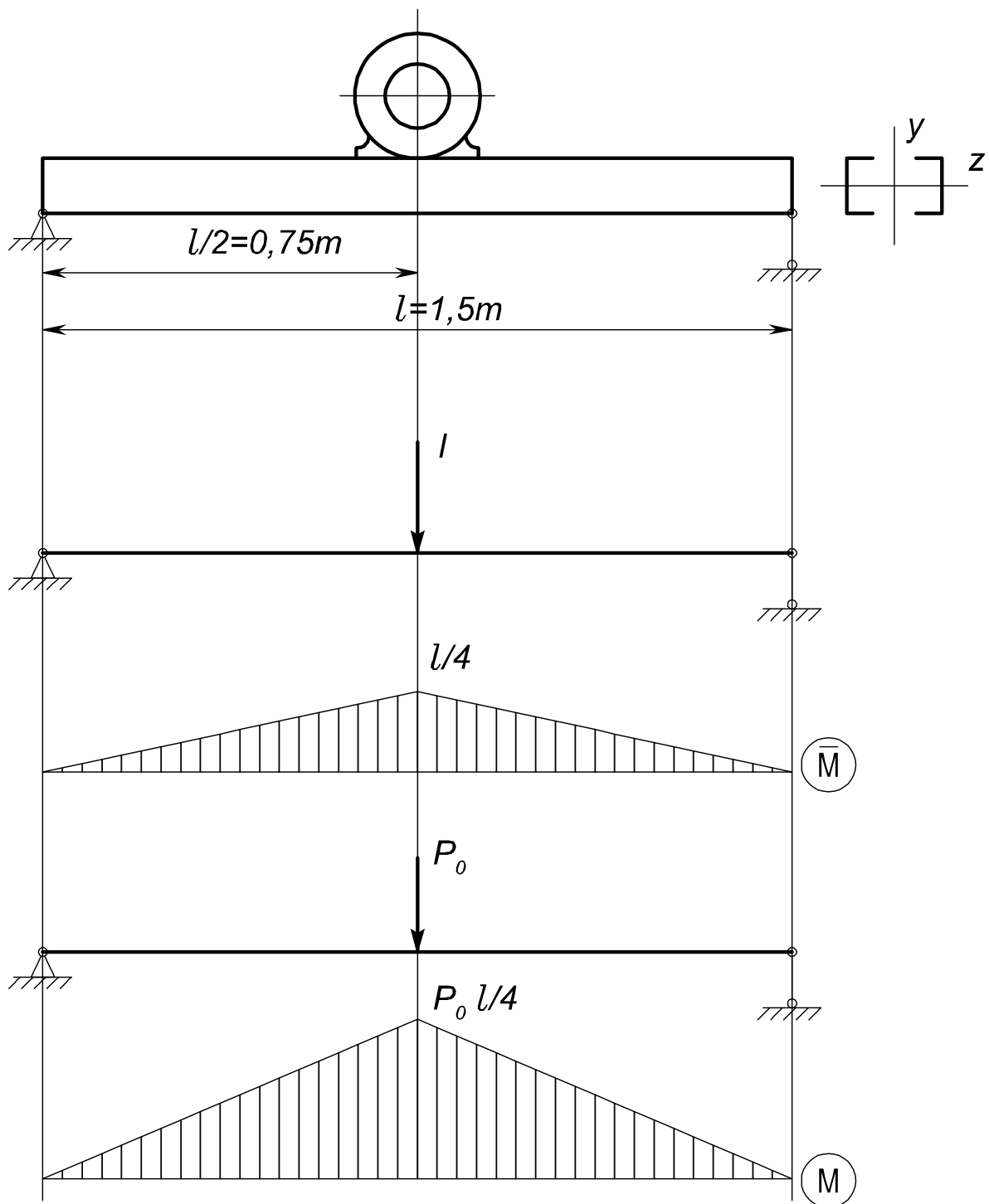
Рис. 1.9. Розрахункова схема навантаження двох балок електродвигуном
