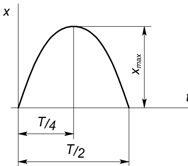
Рис. 4.2. Графік руху приєднаної маси при горизонтальному ударі
