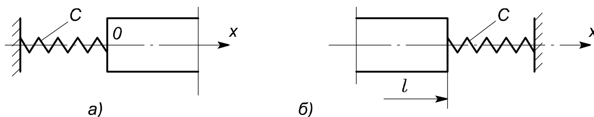
Рис. 2.3. Розрахункові схеми пружних закріплень стрижнів
