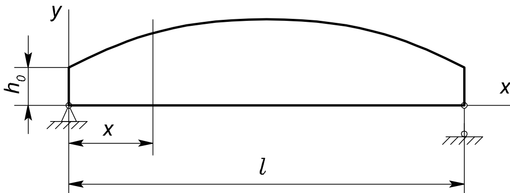
Рис. 3.5. Розрахункова схема двоопорної балки
