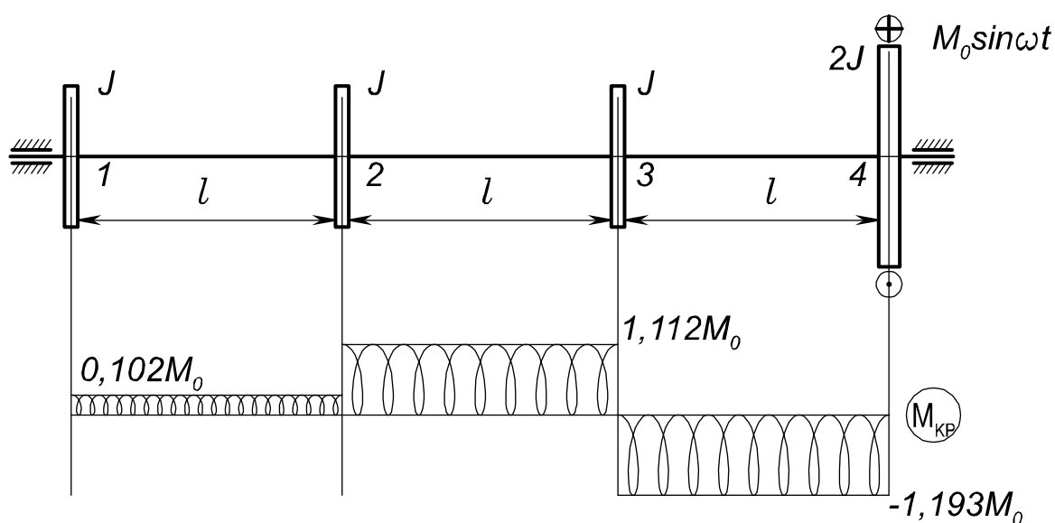
Рис. 1.11. Розрахункова схема чотиримасової крутильної системи
