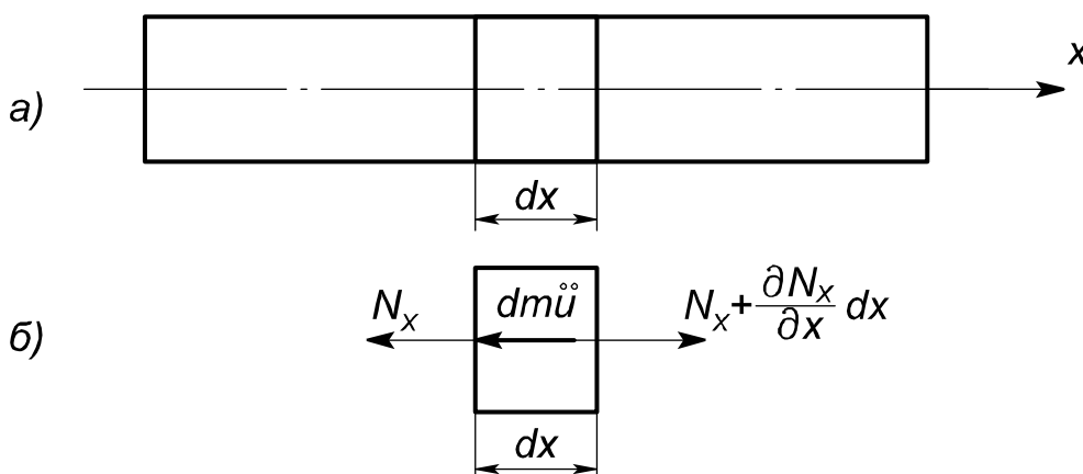
Рис. 2.2. Розрахункова схема стрижня
