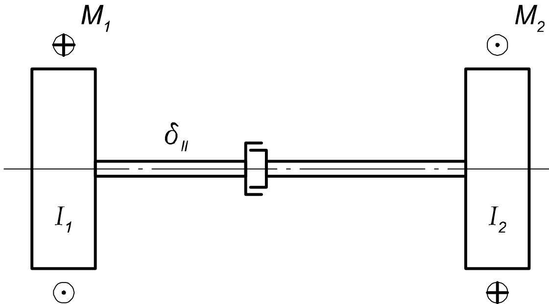
Рис. 5.10. Розрахункова схема двомасової системи з зазором
