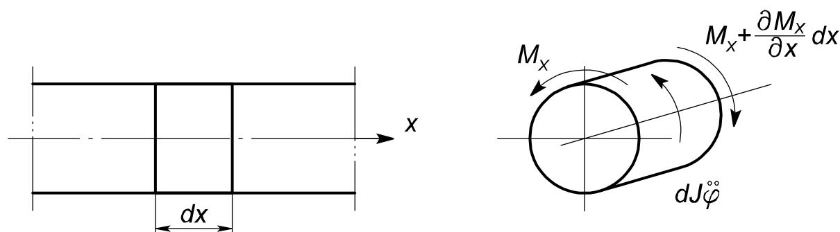
Рис. 2.5. Розрахункова схема вала
