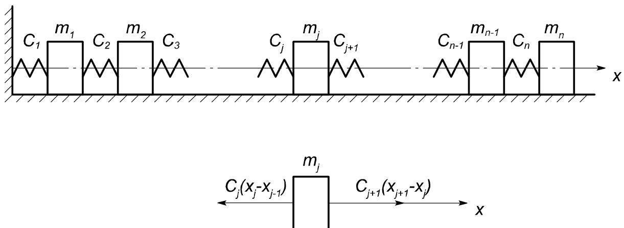
Рис. 1.4. Багатомасова система з пружними елементами, які працюють на розтягнення та стиснення
