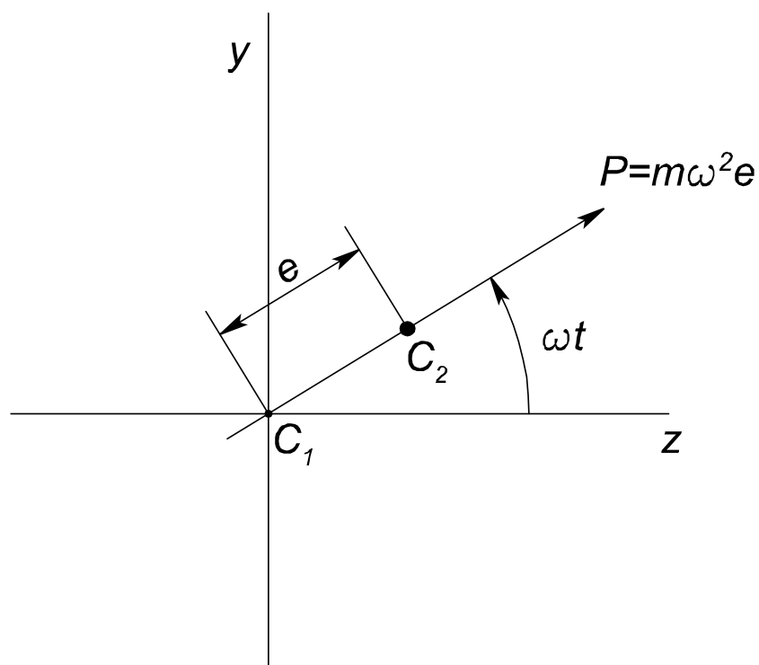
Рис. 5.2. Схема утворення сили дизбалансу вала
