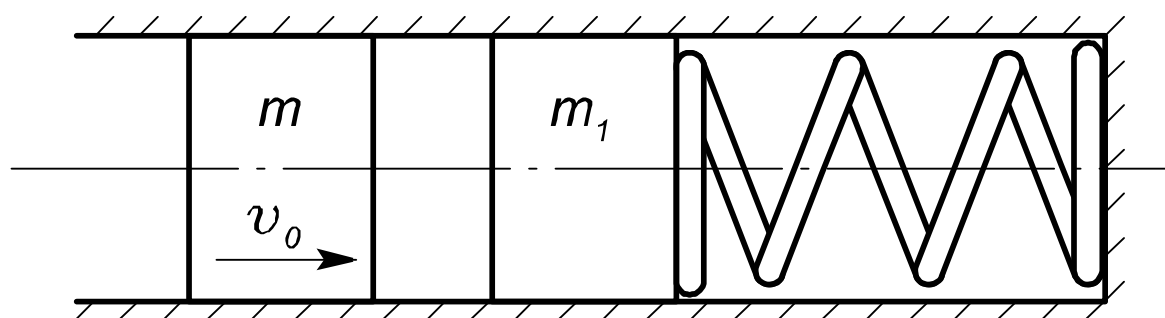
Рис. 4.5. Розрахункова схема системи при поздовжньому ударі з урахуванням проміжної маси
