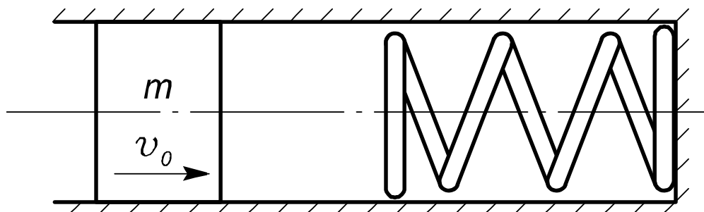
Рис. 4.1. Розрахункова схема системи при поздовжньому ударі
