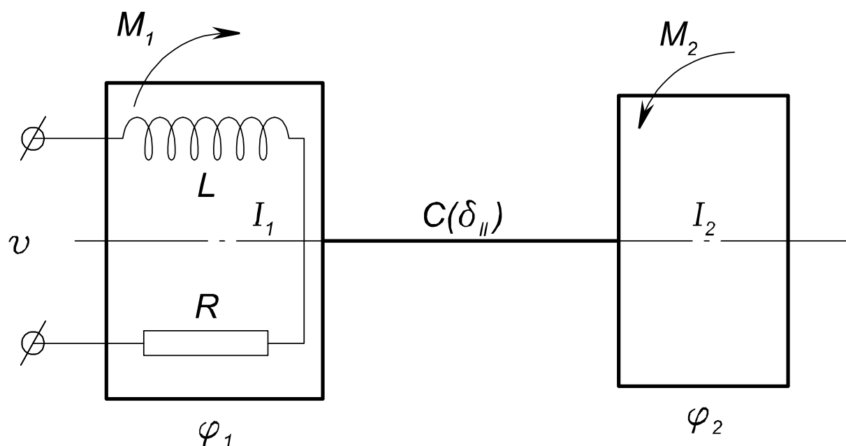
Рис. 5.12. Електромеханічна система привода
