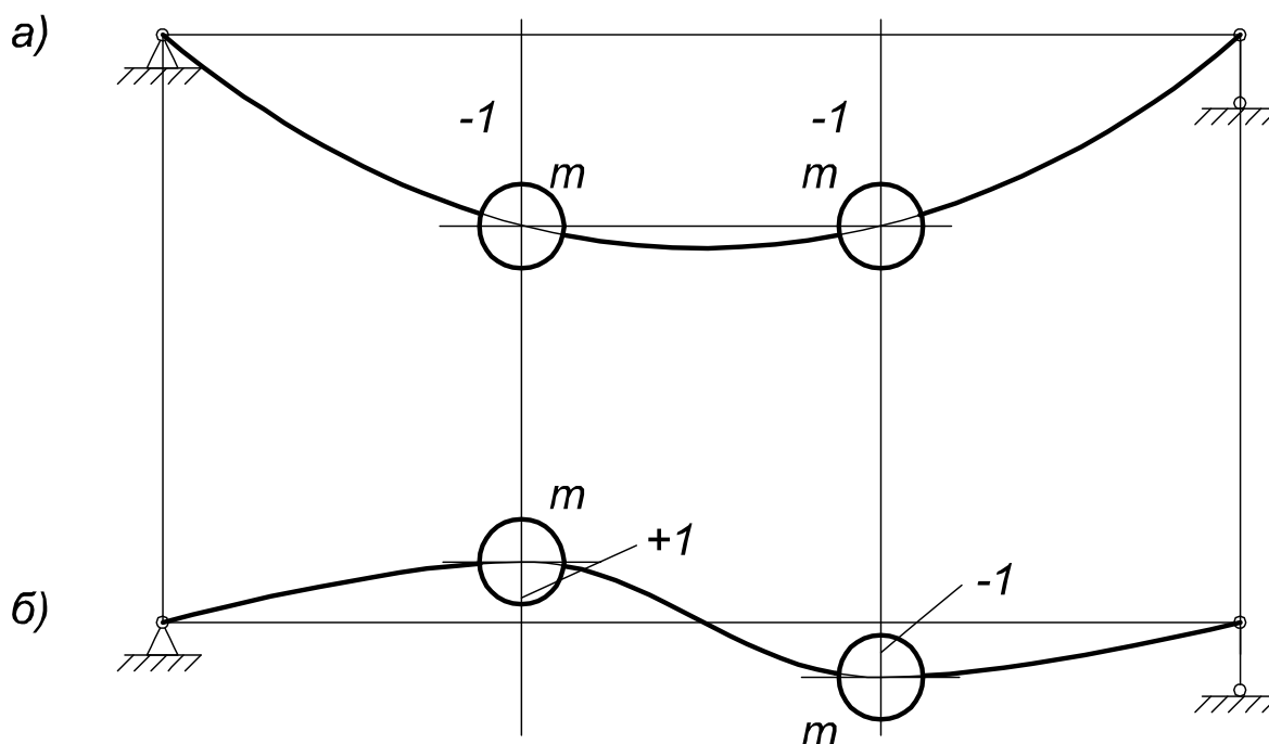
Рис. 1.8. Власні форми коливань двомасової балочної системи
