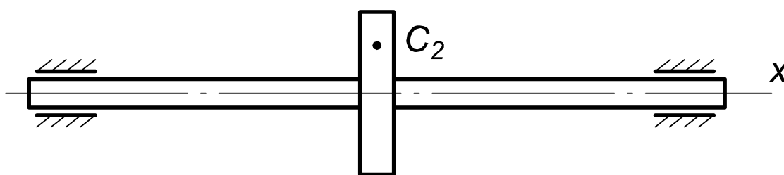
Рис. 5.1. Розрахункова схема вала з диском
