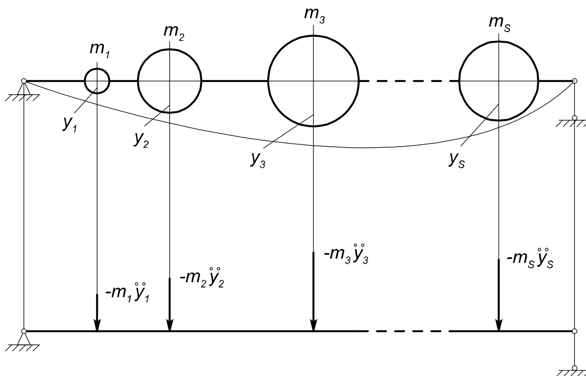
Рис. 1.6. Багатомасова балочна система
