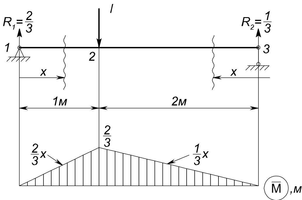
Рис. 5.6. Епюра згинаючих моментів
