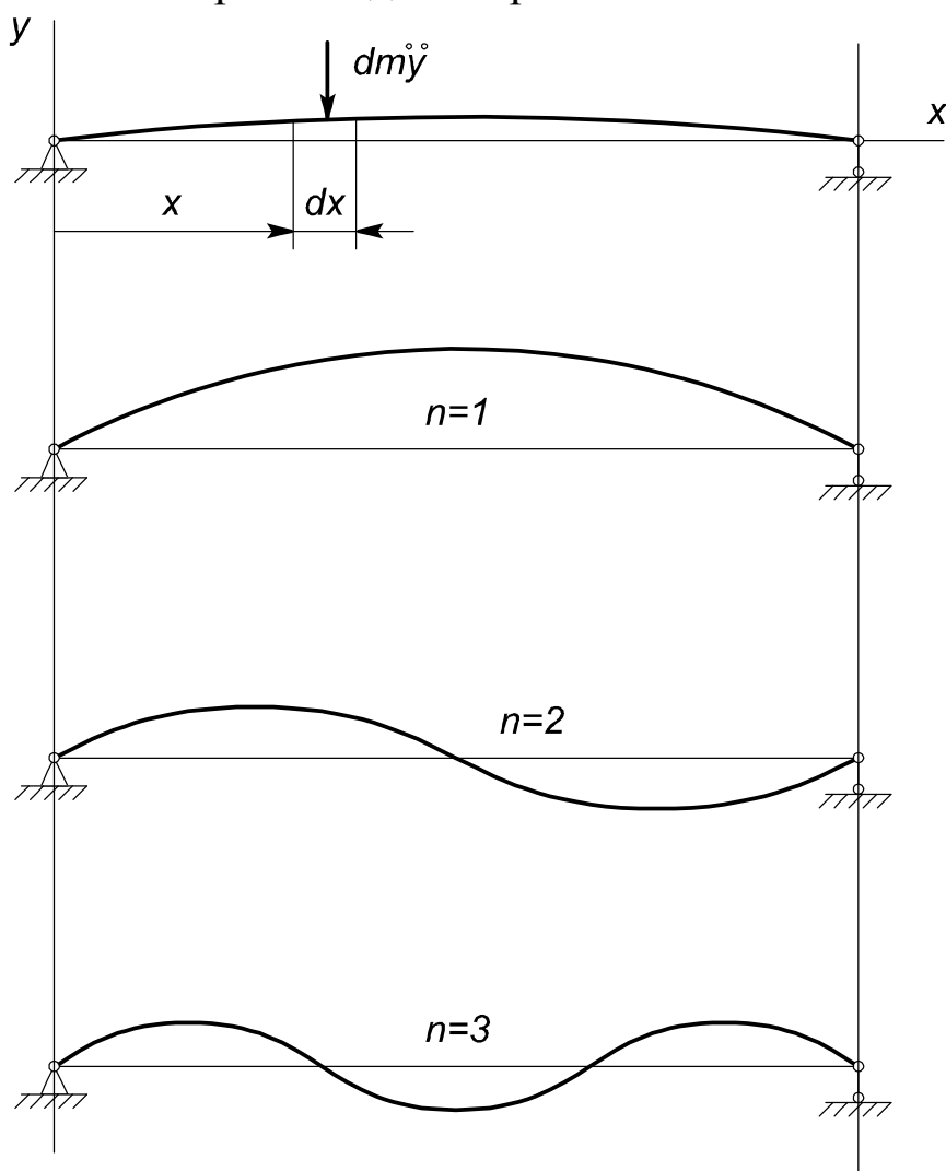
Рис. 2.8. Розрахункова схема та форми коливань двоопорної балки
