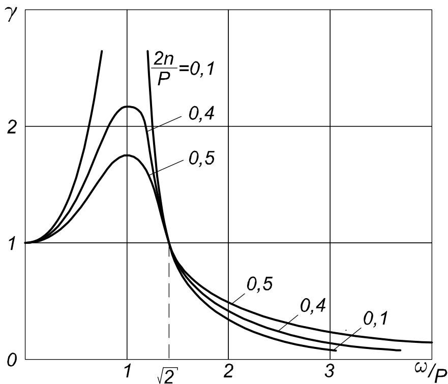
Рис. 5.8. Графіки залежності коефіцієнта віброізоляції \gamma від відношення \omega/p
