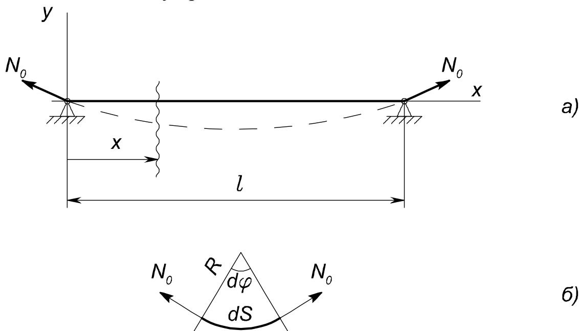
Рис. 2.1. Розрахункова схема струни
