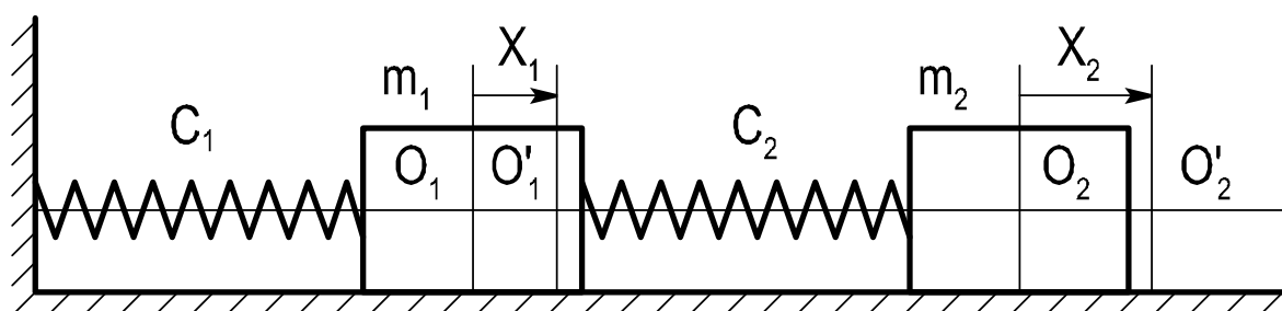
Рис. 1.1. Розрахункова схема двомасової системи до основного способу
