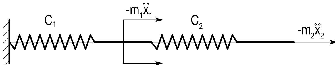
Рис. 1.3. Розрахункова схема двомасової системи до оберненого способу
