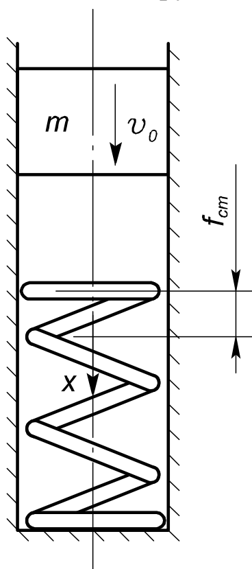
Рис. 4.3. Розрахункова схема системи при вертикальному поздовжньому ударі
