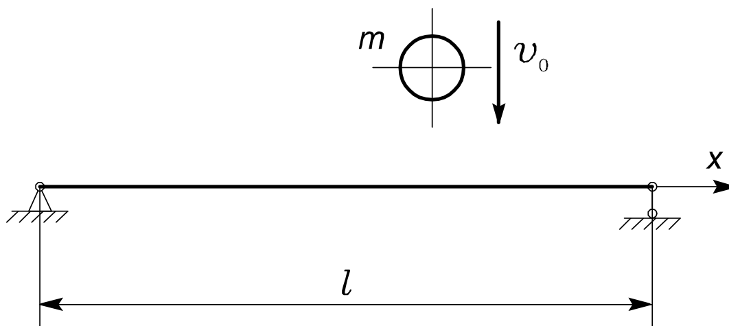
Рис. 4.7. Розрахункова схема балки
