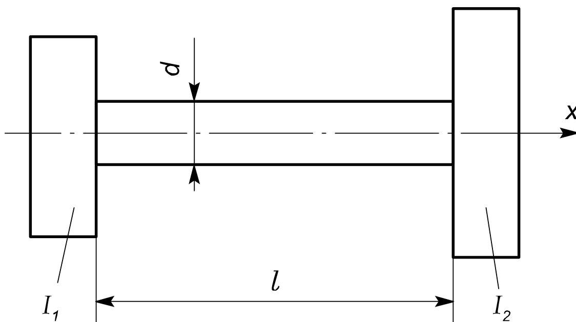
Рис. 2.7. Розрахункова схема вала з двома дисками
