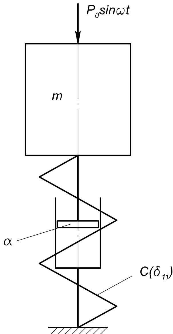
Рис. 5.7. Розрахункова схема активної віброізоляції Рівняння коливань такої системи має наступний вигляд:
