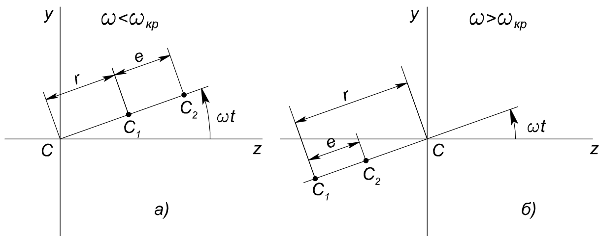
Рис. 5.3. Розташування характерних точок вала в залежності від співвідношення \omega/p .
