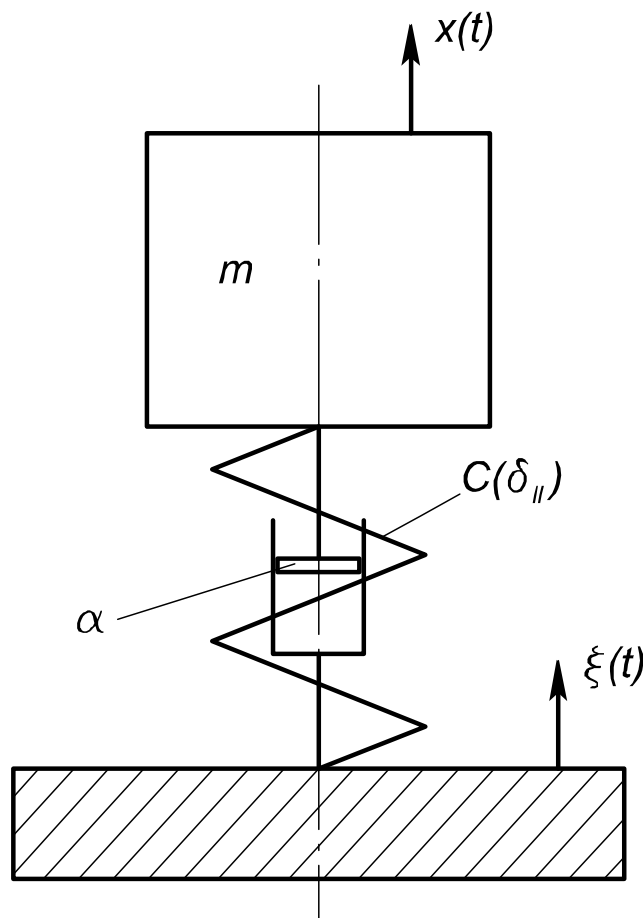
Рис. 5.9. Розрахункова схема пасивної віброізоляції
