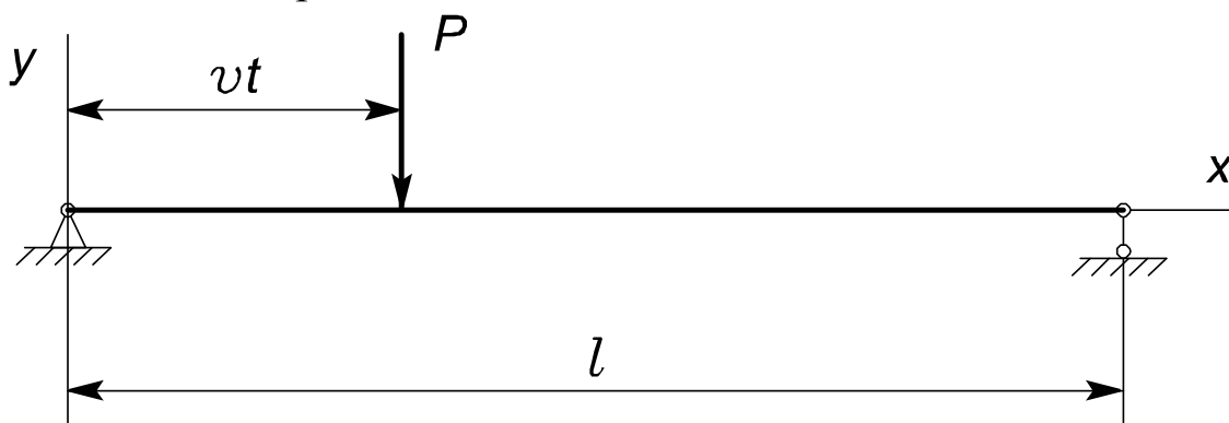
Рис. 2.9. Розрахункова схема балки з рухомою постійною силою
