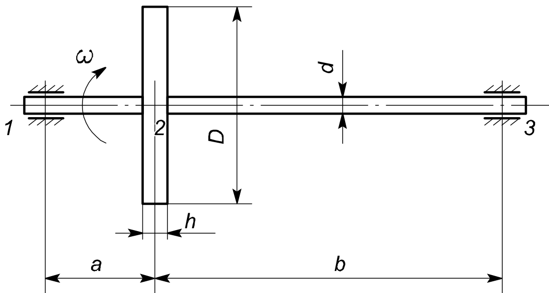
Рис. 5.5. Розрахункова схема вала з диском.
